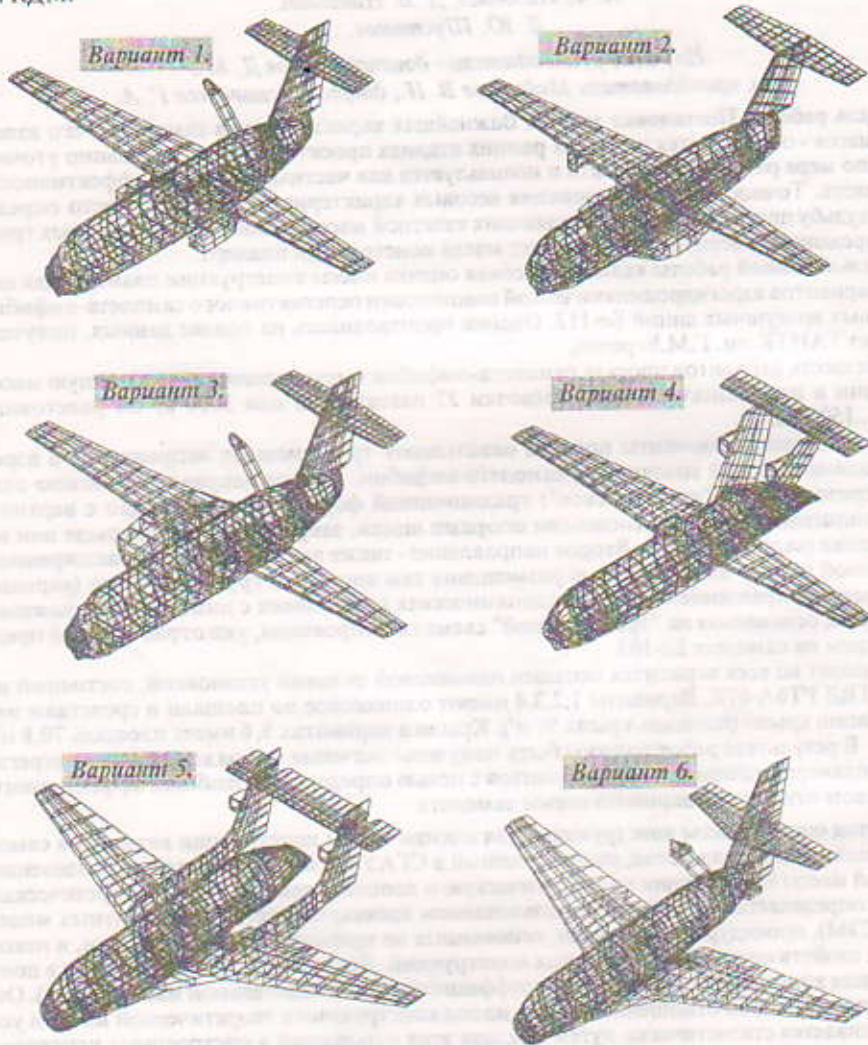
Рис. 1. КЭМ вариантов самолета
